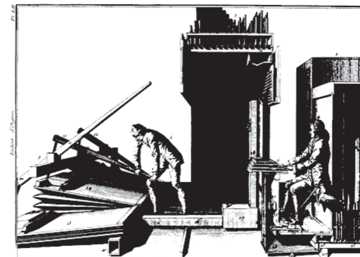
27 Schnitt durch die französische Orgel des 18. Jahrhunderts nach Dom Bédos de Celles. (L'art du facteur d'orgues, Paris 1766 ff., Tafel L.II.)
